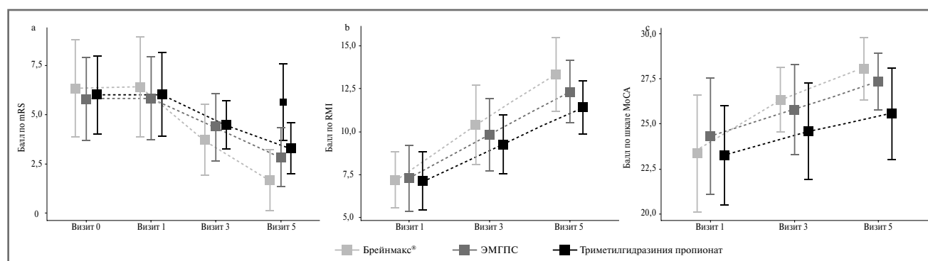
Рис. 4. Динамика среднего суммарного балла по NIHSS (a), среднего суммарного балла по RMI (b), среднего суммарного балла по шкале MoCA (c).
