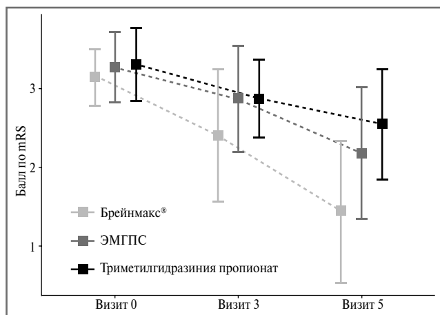
Рис. 3. Суммарная динамика баллов по mRS.
